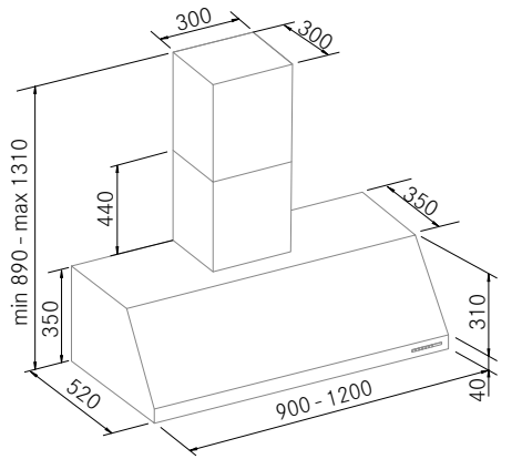
Diseño técnico Tubo Salida 150 mm.
