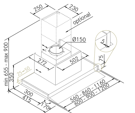
Diseño técnico Tubo Salida 150 mm.
