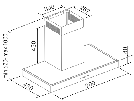
Diseño técnico Tubo Salida ø150 mm. (Medidas exteriores)
