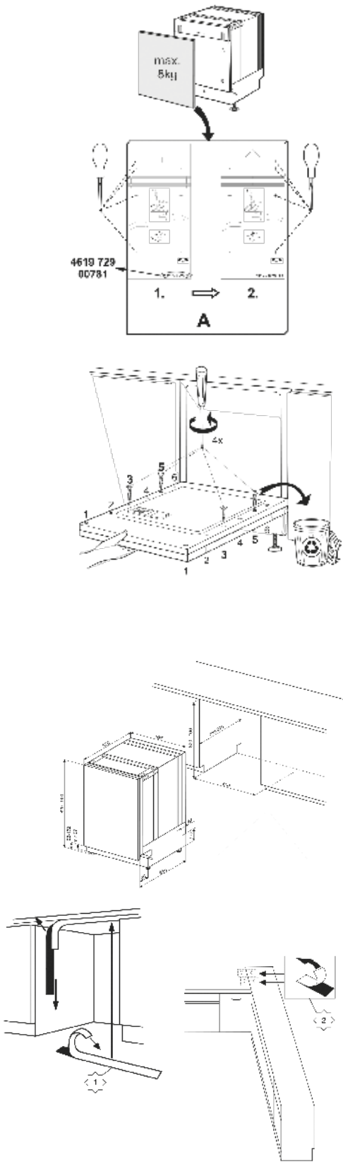
Instalación puerta fija:
